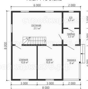
План 1-го этажа
