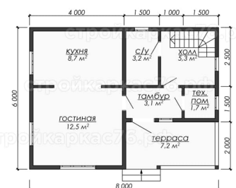
План 1-го этажа
