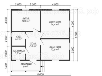
План 1-го этажа
