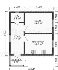
План 1-го этажа
